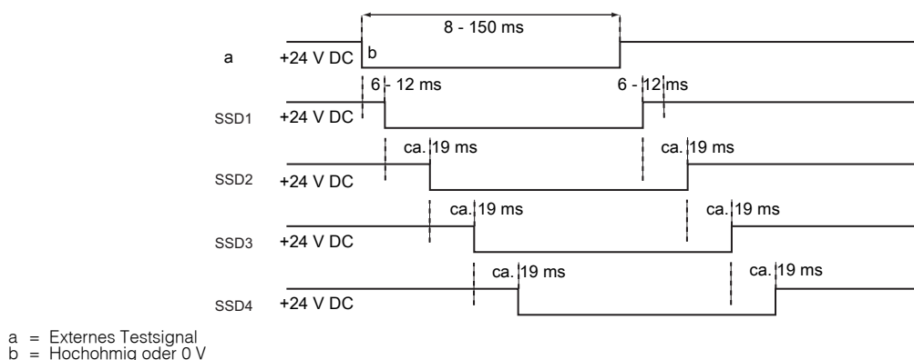
Bild 6.2: Externe Testung SOLID-2SF
