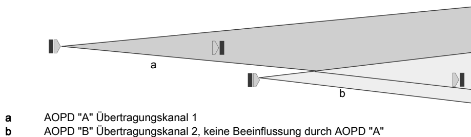
Bild 3.2: Auswahl Übertragungskanal (AOPD = Aktive opto-elektronische Schutzeinrichtung (Active Opto-electronic Protective Device))
