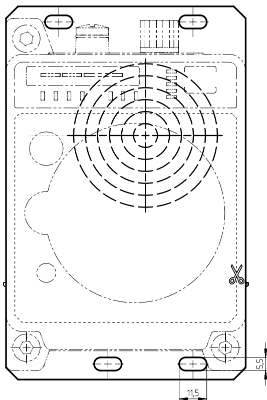
Figura 4.2: Maschera di foratura
