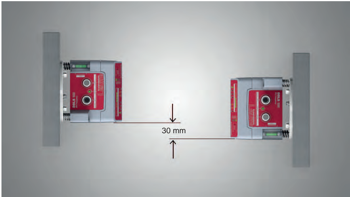
Figura 4.9: Montaggio ad alloggiamenti sfalsati
