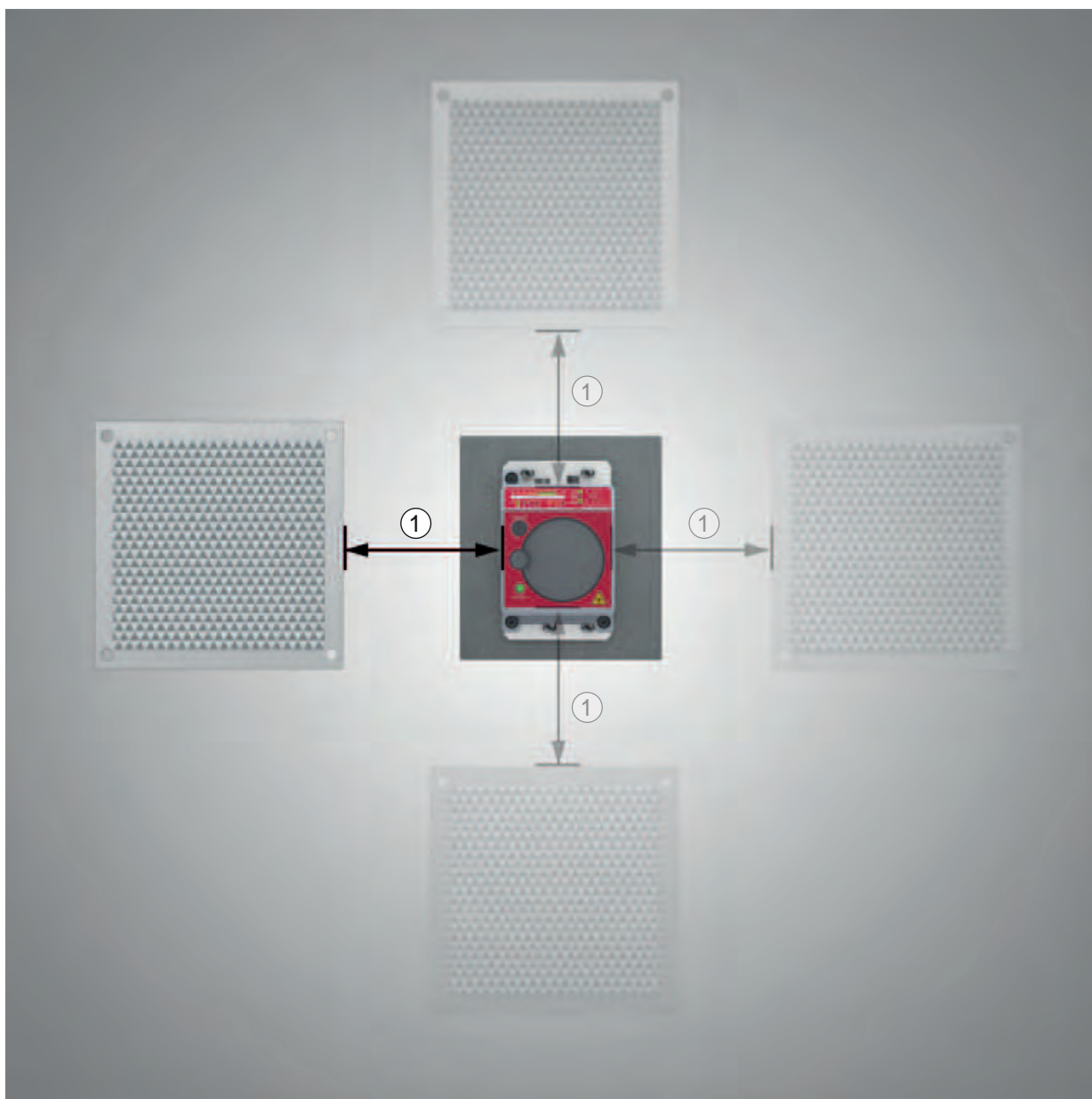
Figura 4.14: Distanza di montaggio minima dal riflettore
