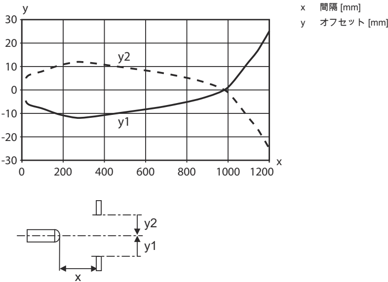
典型的応答挙動 ( 調整距離 1200mm )
