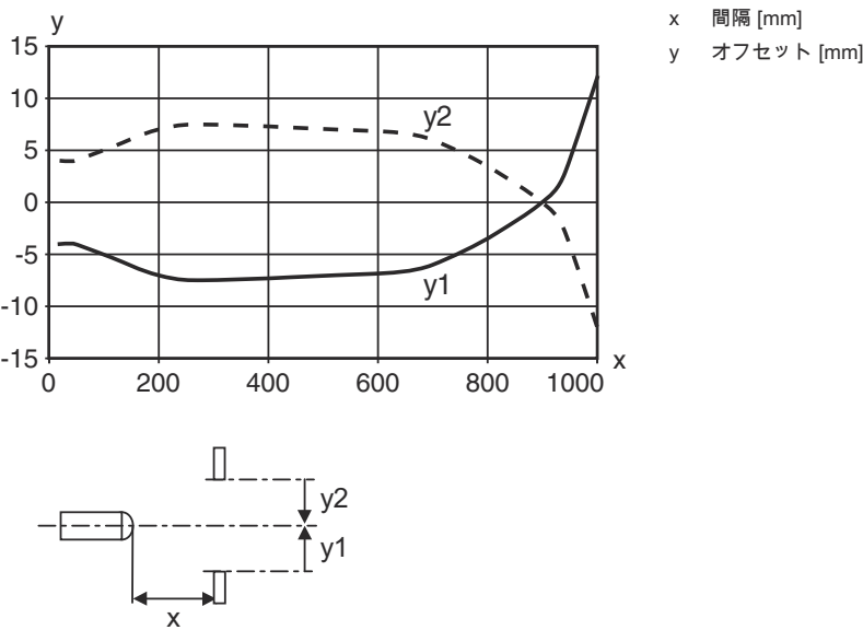
典型的応答挙動 ( 調整距離 1000mm )
