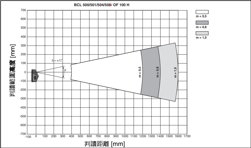
圖 5.26：含加熱之振鏡式掃描器的側向「低密度」判讀範圍曲線
