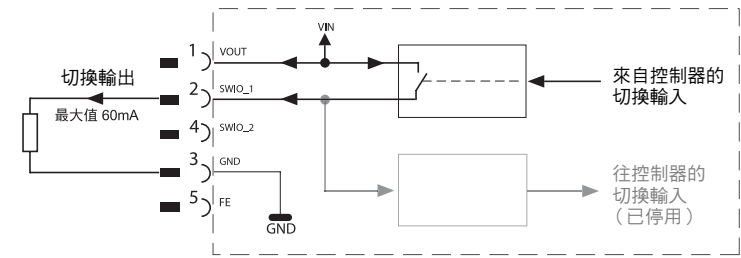
圖 7.6： SWIO_1 / SWIO_2 切換輸出連接順序圖
