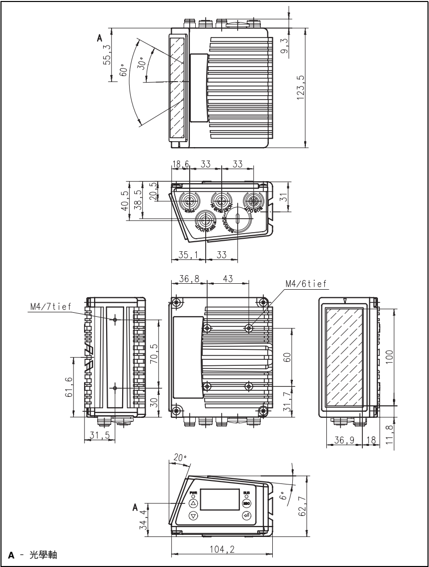
圖 5.1 : BCL 504 i 線式掃描器 S...102 外觀尺寸圖
