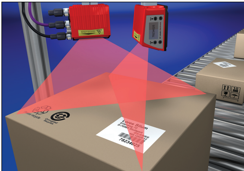
圖 4.6：全方位判讀的原理佈置
