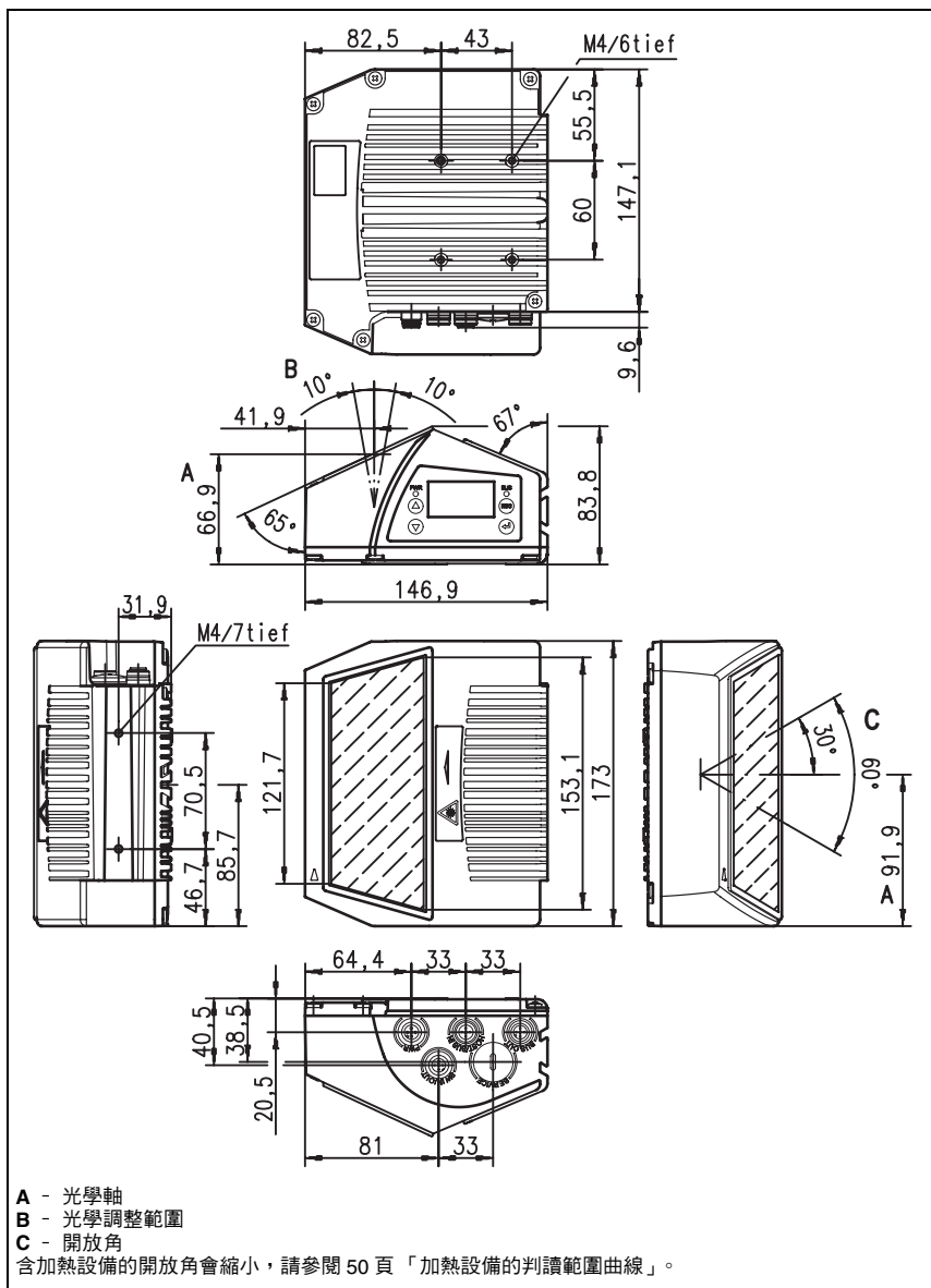
圖 5.2： BCL 504 i 偏鏡式掃描器 S...100 外觀尺寸圖
