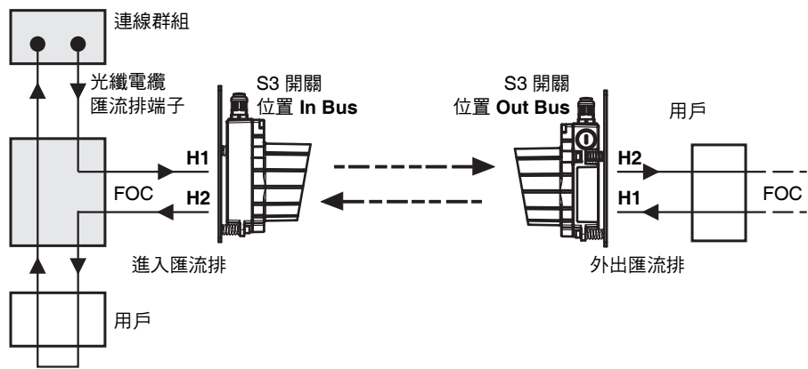
圖 7.2： DDLS 200 到 INTERBUS 的连接（光纖電纜）
