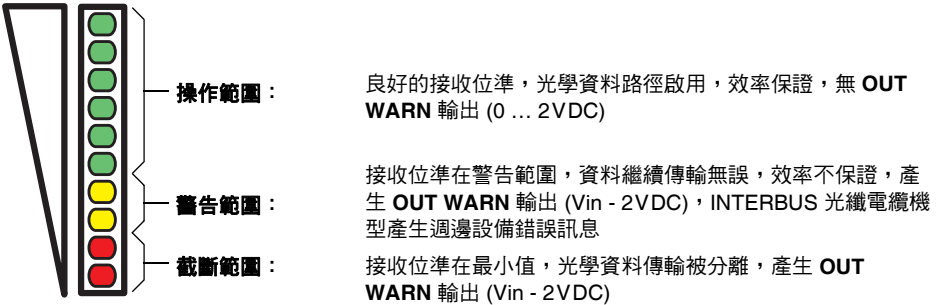
圖 11.2：用來顯示接收位準之長條燈號的意義
