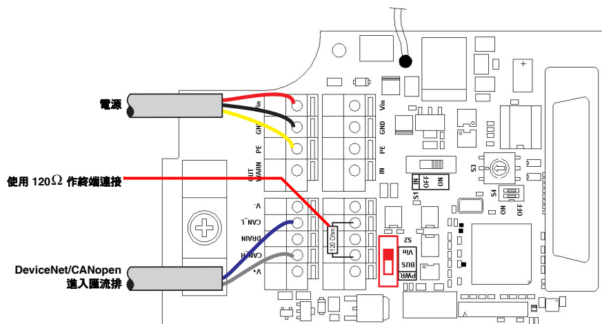
圖 9.10：設備內的終端連接。
