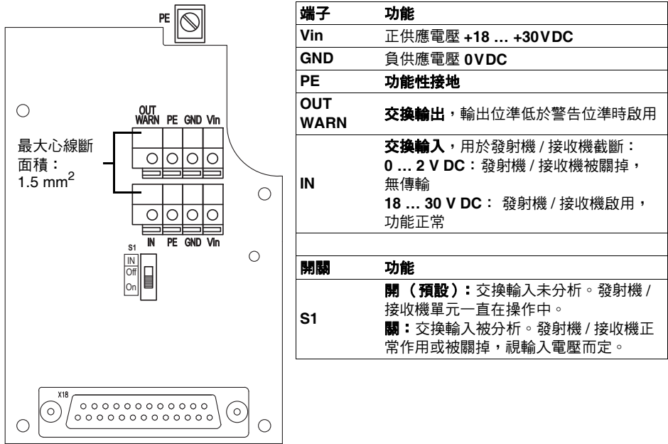
圖 4.5：通用、非特定匯流排專用端子以及開關的位置
