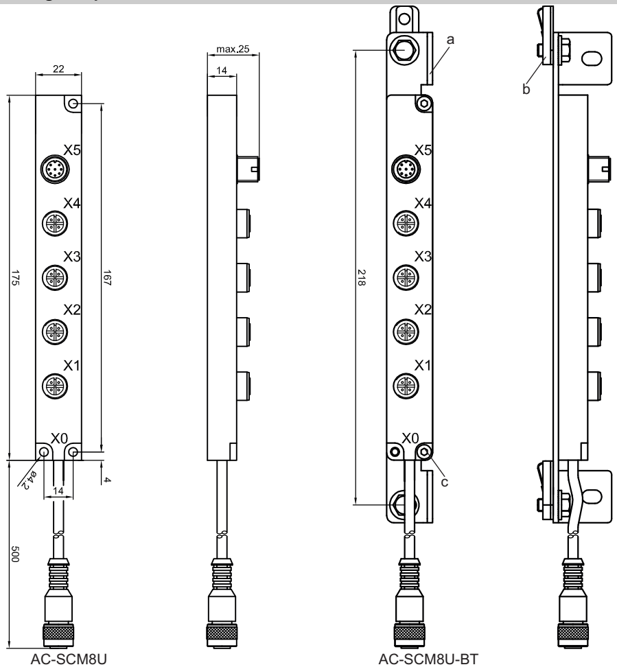
a = piastra di montaggio b = tassello scorrevole c = viti a testa cilindrica M4x16
