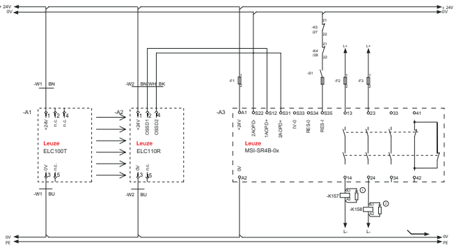
带后置安全控制器MSI-SR4B的接线示例
