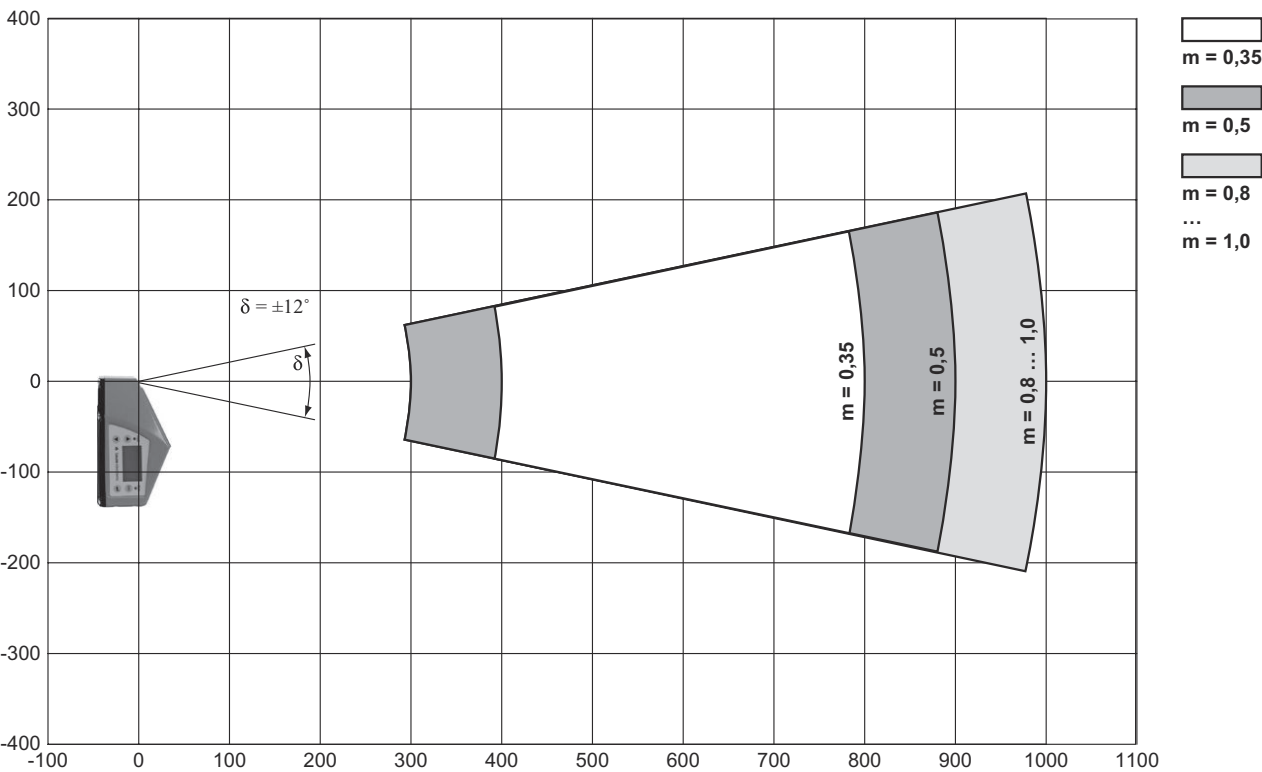
측방향 판독 필드 커브
