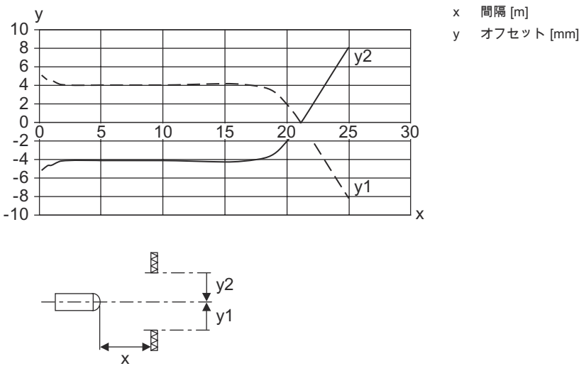
典型的な応答動作 ( TKS100x100 )
