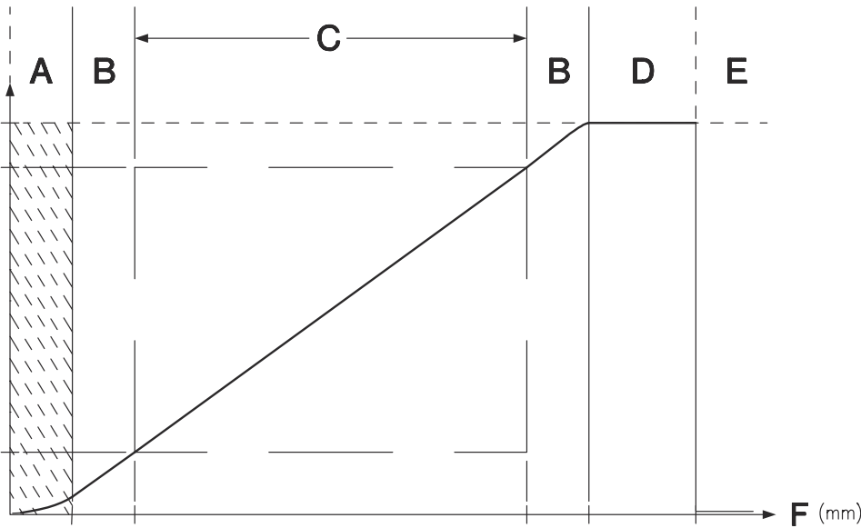
模拟输出端输出特性曲线
