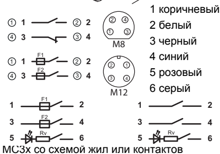
MC3x со схемой жил или контактов
