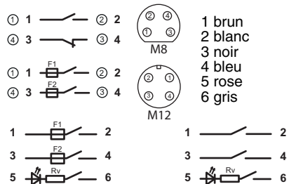
MC3x avec câblage ou brochage
