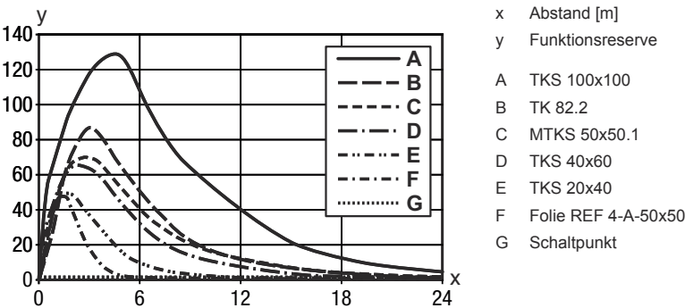
Typ. Funktionsreserve
